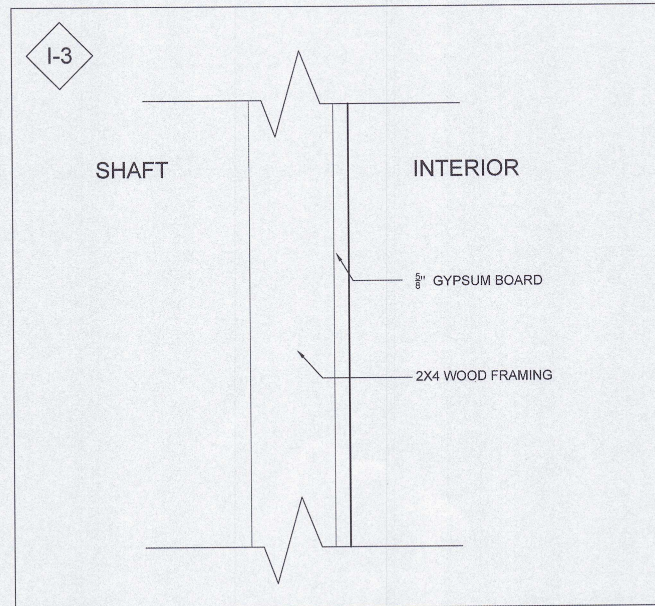
6 INTERIOR 2X4 SHAFT WALL SCALE: 3" = 1'-0"
