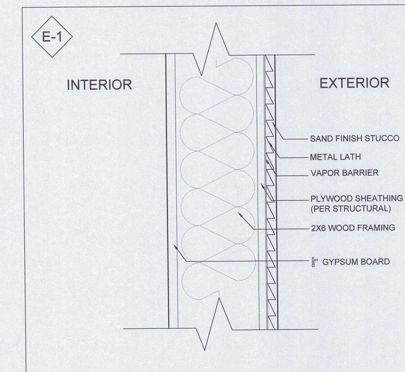
1 TYP EXTERIOR 2X6 WALL SCALE: 3" = 1'-0"
