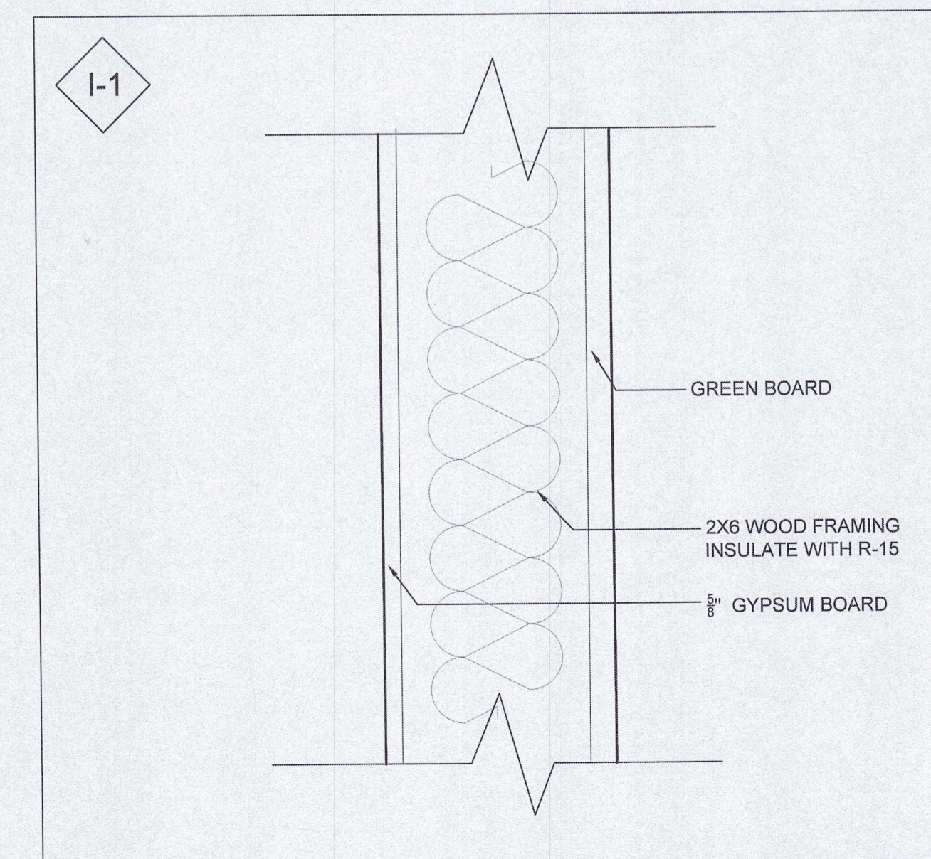
4 INTERIOR 2X6 PLUMBING WALL SCALE: 3" = 1'-0"
