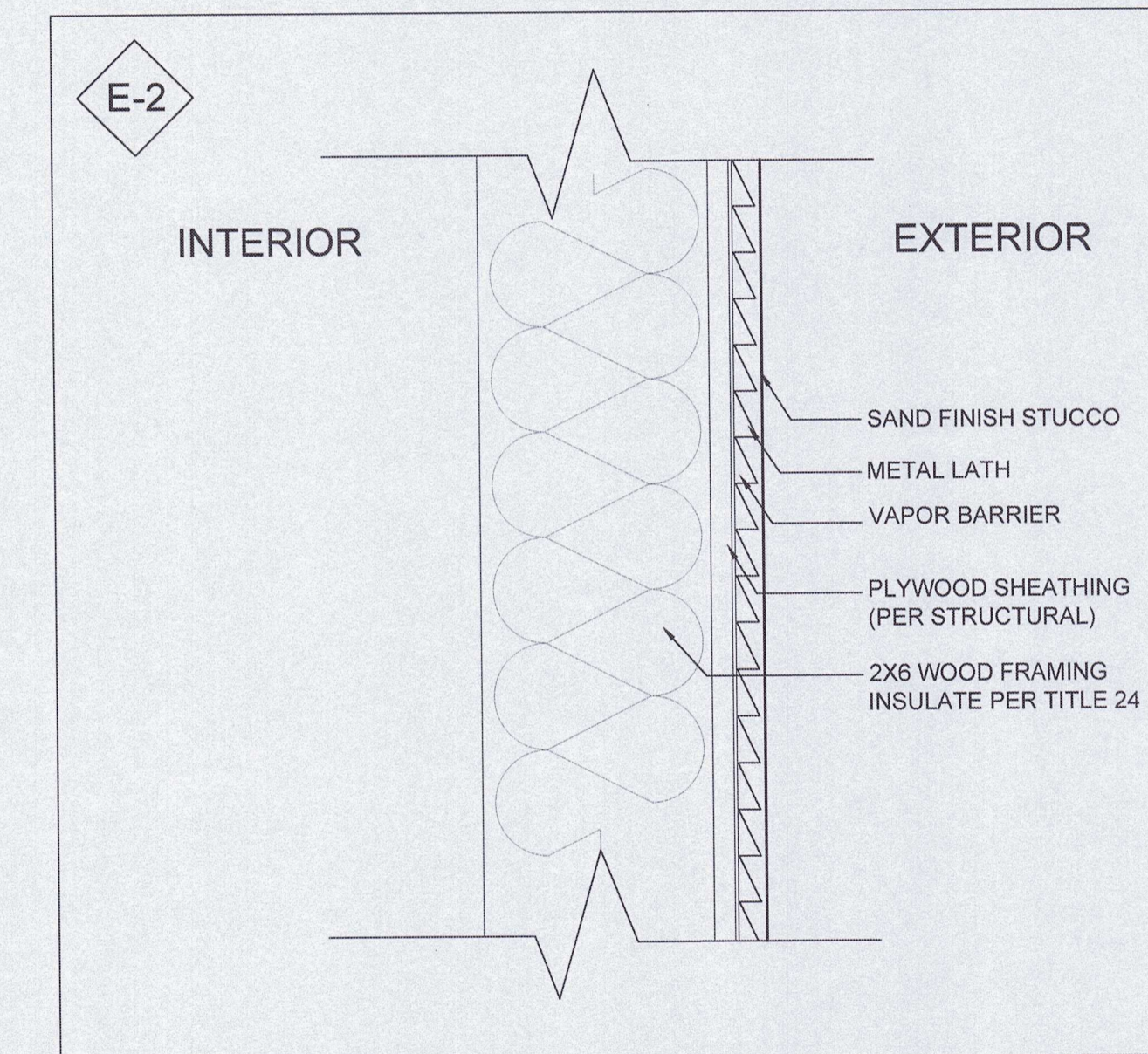
2 EXTERIOR 2X6 SHAFT WALL SCALE: 3" = 1'-0"
