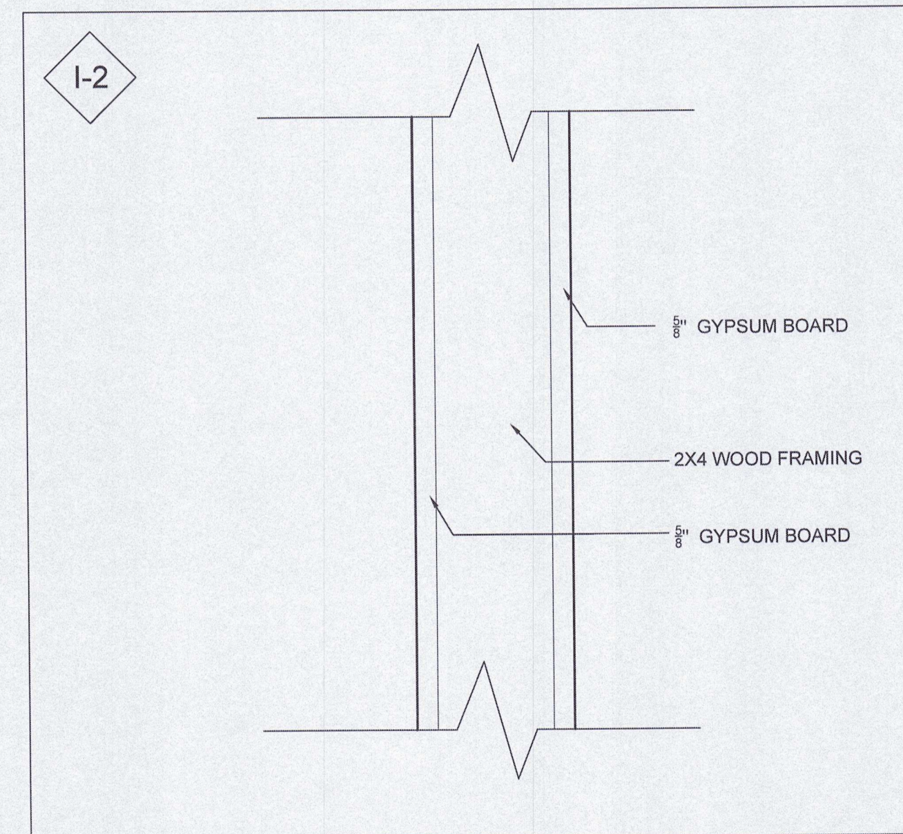
5 INTERIOR 2X4 WALL SCALE: 3" = 1'-0"
