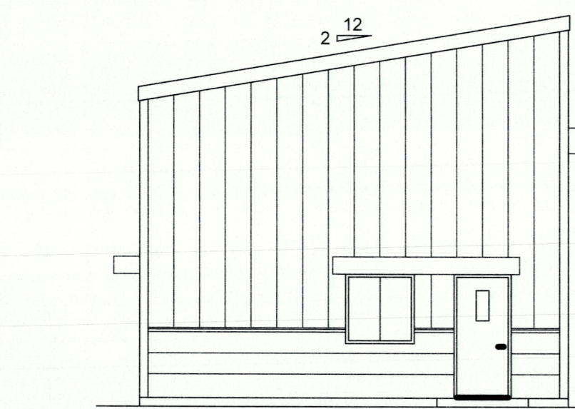
BLDG 'C': REAR SCALE: 1/8"=1'-0"
