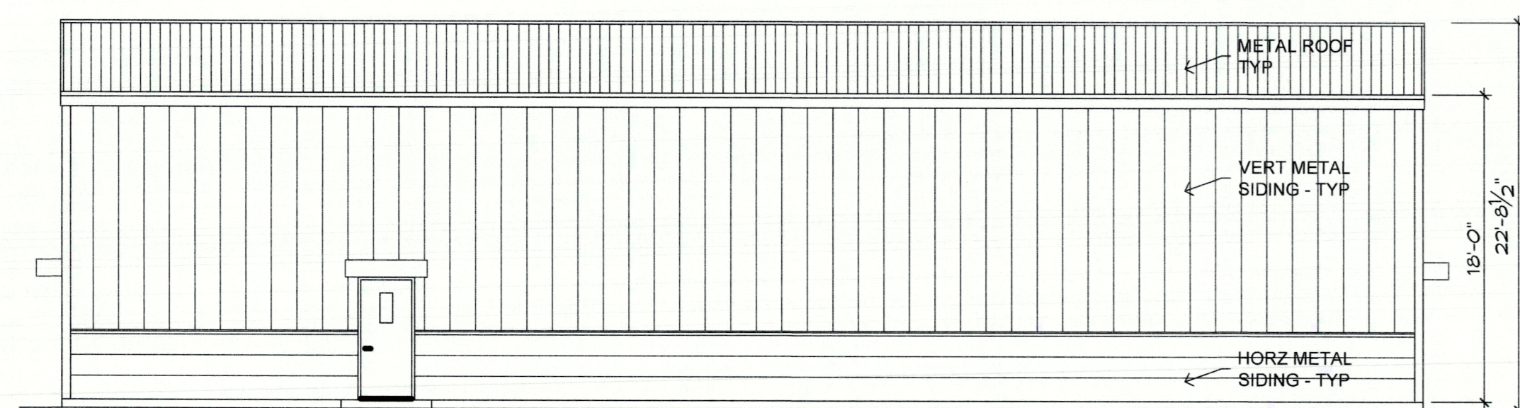
BLDG 'C': REAR SCALE: 1/8"=1'-0"
