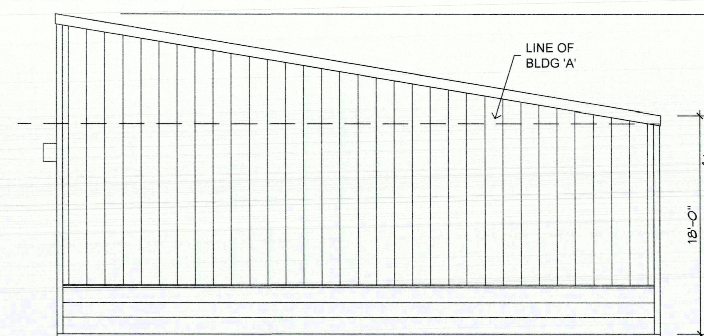
BLDG 'B': SIDE SCALE: 1/8"=1'-0"
