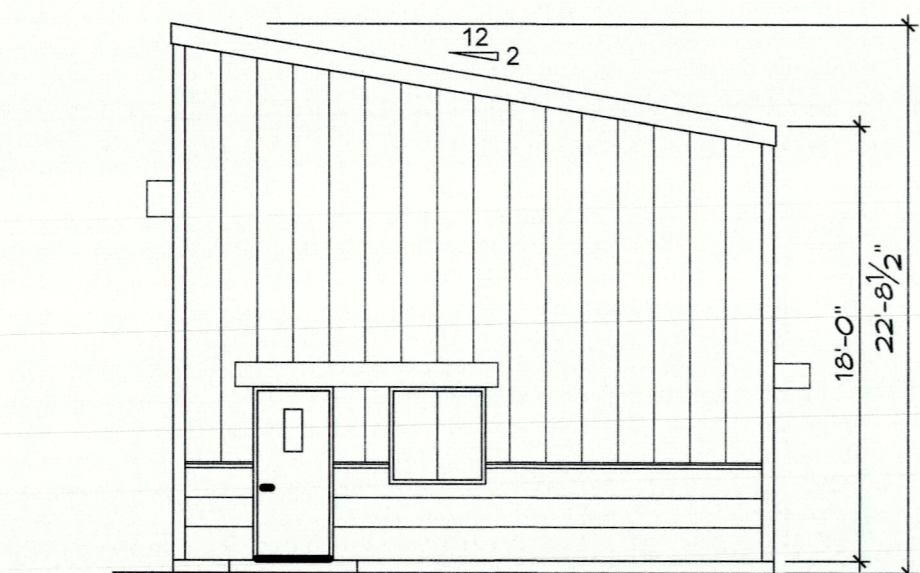
BLDG 'C': REAR SCALE: 1/8"=1'-0"
